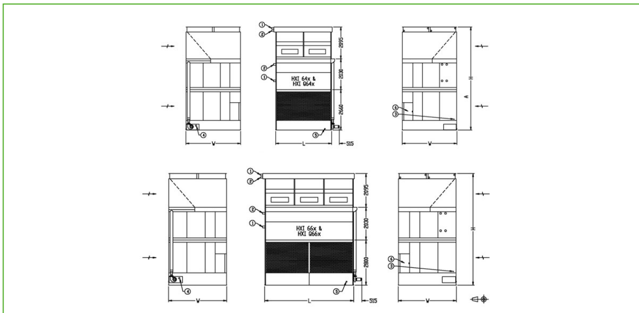
1. Впускное соединение; 2. Выпускное соединение; 3. Подпитка НД 25; 4. Перелив НД 80; 5. Слив НД 50; 6. Дверца люка.
