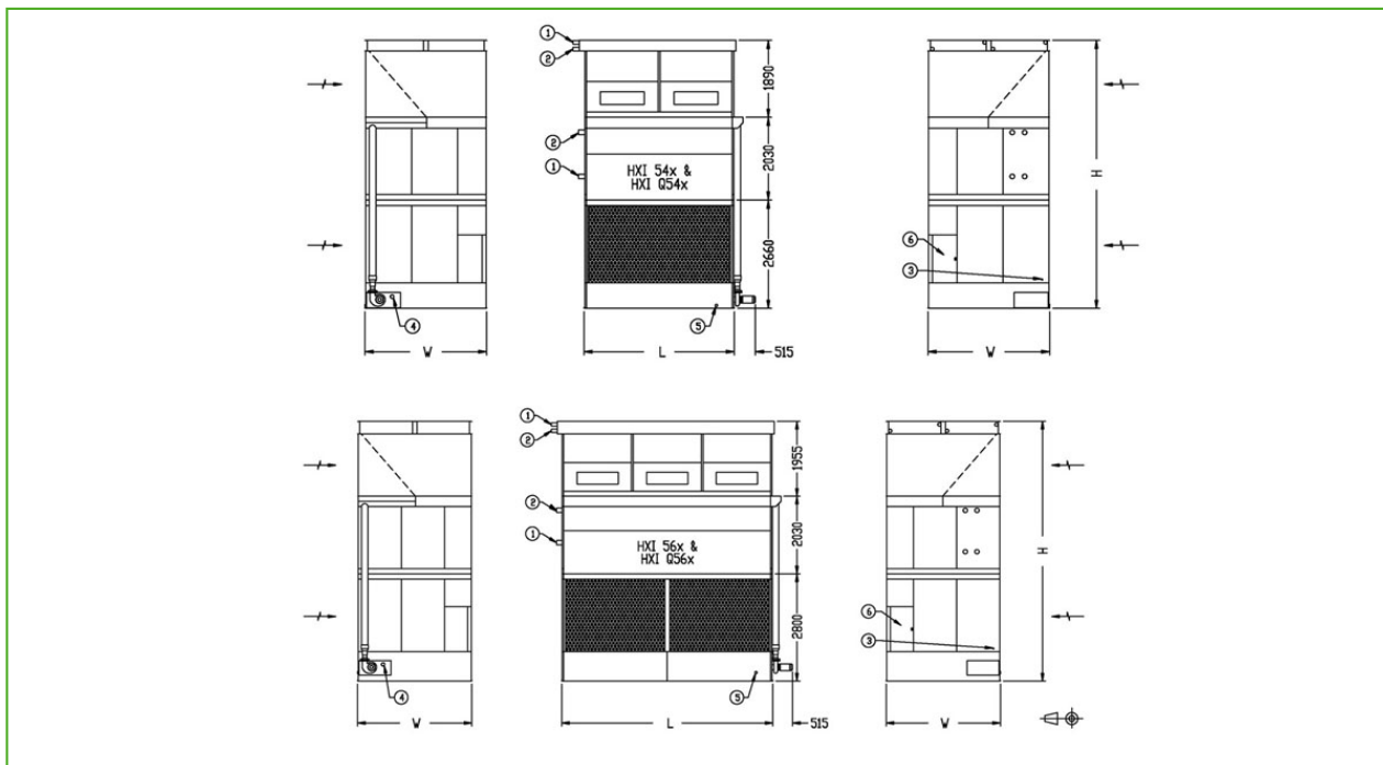
1. Впускное соединение; 2. Выпускное соединение; 3. Подпитка НД 25; 4. Перелив НД 80; 5. Слив НД 50; 6. Дверца люка.
